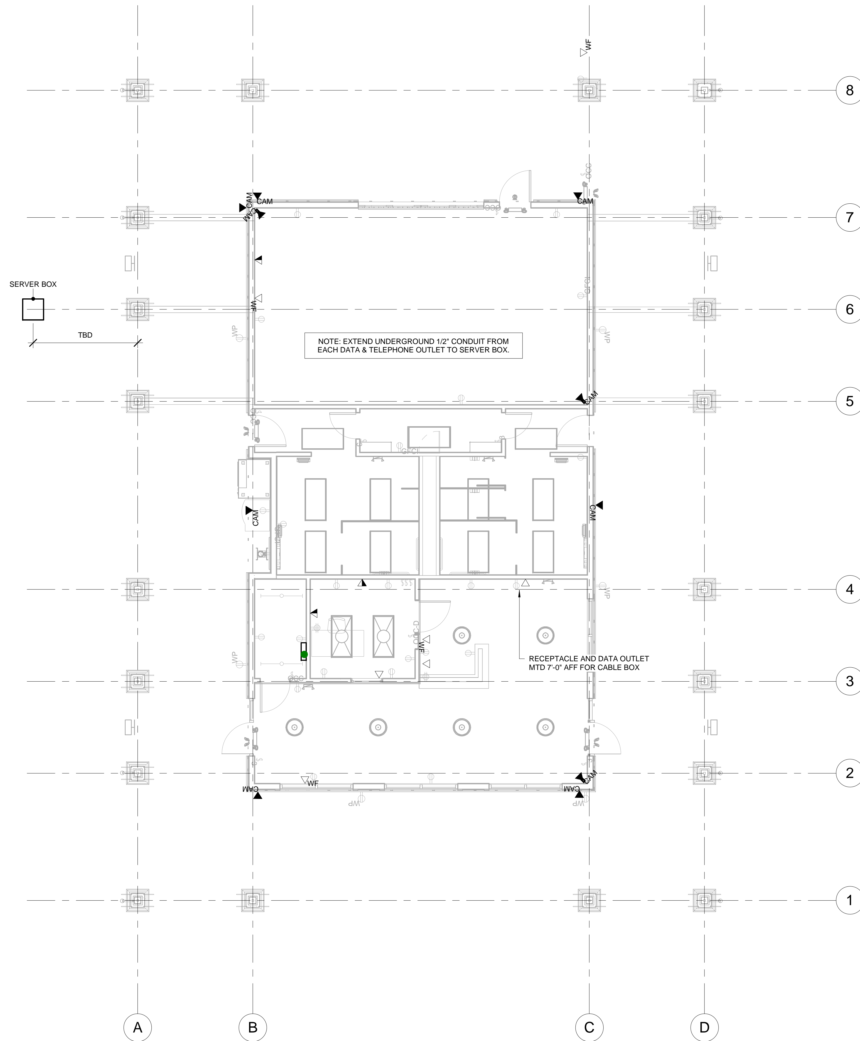
1 - DATA-COMM SCALE: 3/16" = 1'-0"
