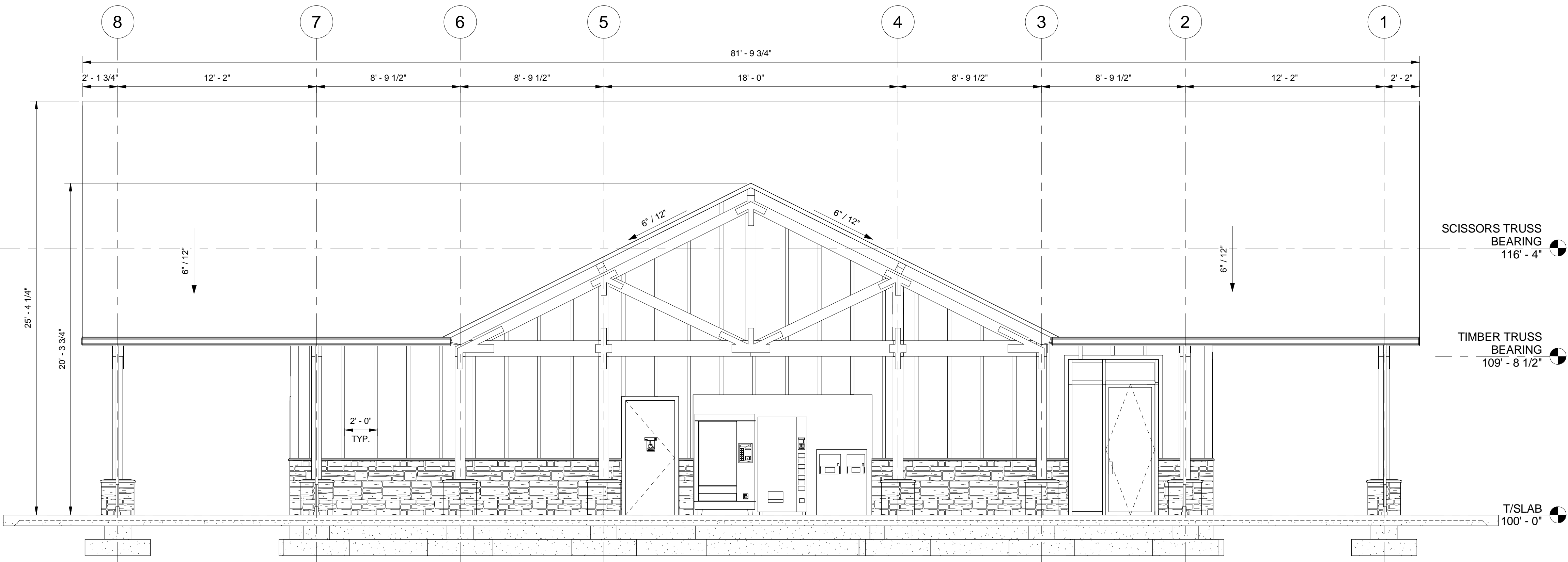
1 NORTH SCALE: 1/4" = 1'-0"
