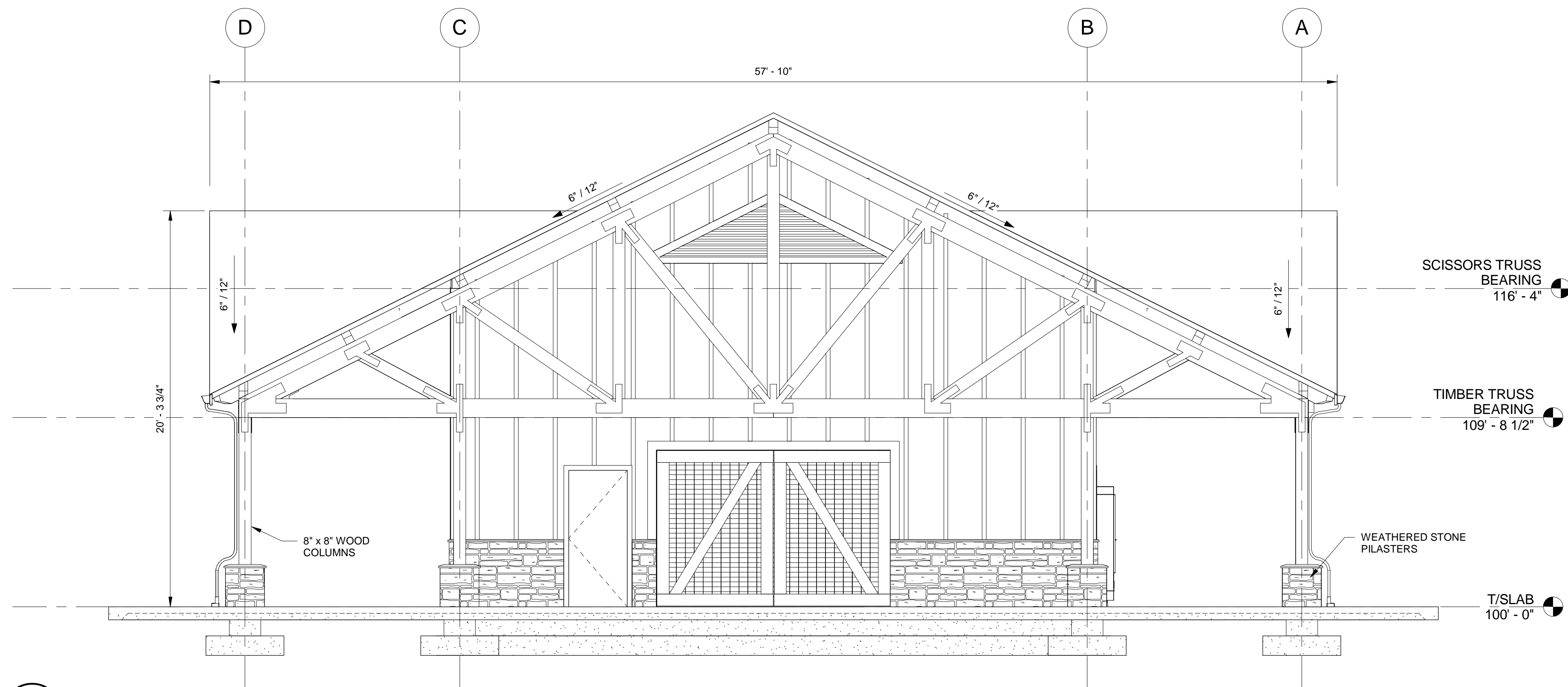
2 WEST SCALE: 1/4" = 1'-0"
